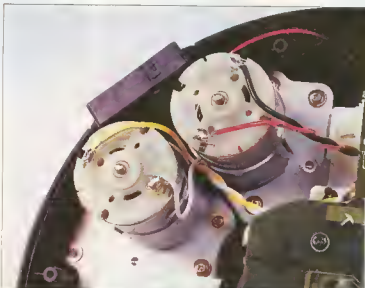
Das Innenleben: Deutlich erkennbar sind die zwei Elektromotoren für die X- und Y-Achse.
